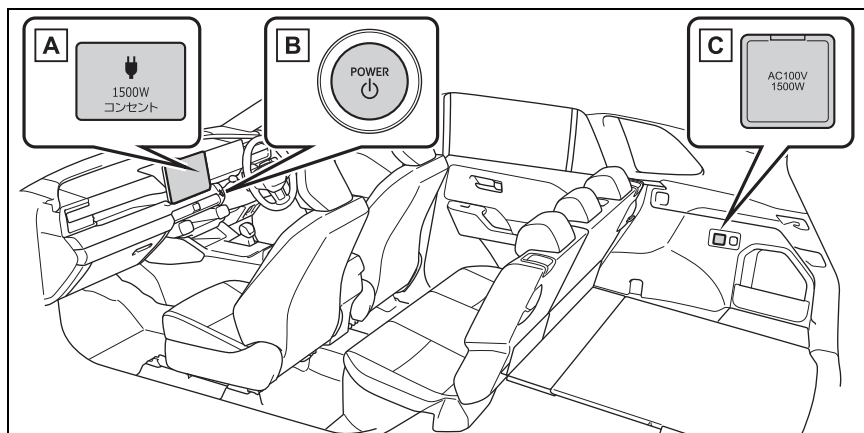
A “1500W コンセント” スイッチ
