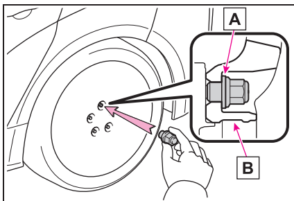
A 座金
