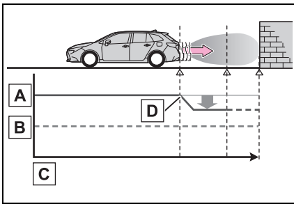
● 図 2 (ハイブリッドシステム出力抑制制御時)
