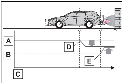
Ⅰ 図 3 (EV システム出力抑制制御 かつブレーキ制御時)
