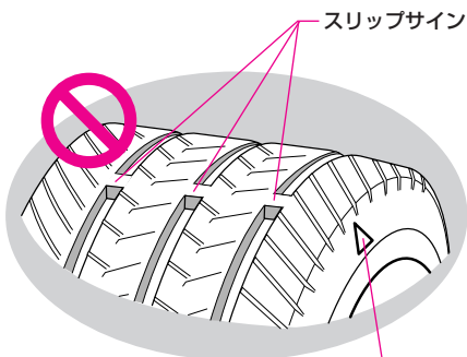
スリップサインの位置を示すマーク
