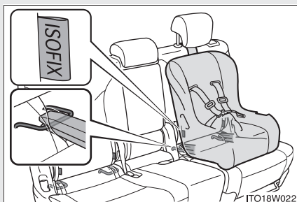
ISOFIX 対応チャイルドシート 固定専用バー (→P. 132)
