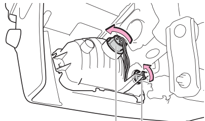
制動灯/尾灯 後面方向指示灯 兼非常点滅灯
