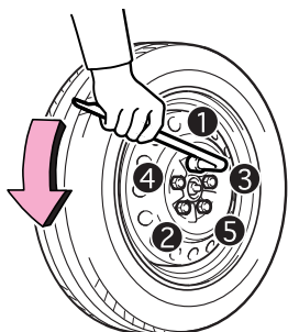
ホイールナットレンチ
