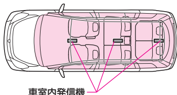
車室内発信機
