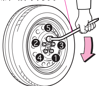
ホイールナットレンチ
