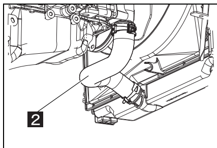
2 ラジエーターロアホース
