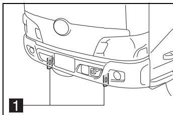
1 輸送用フック
