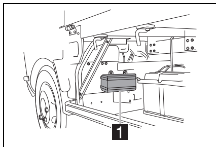
1 室外ヒューズボックス
