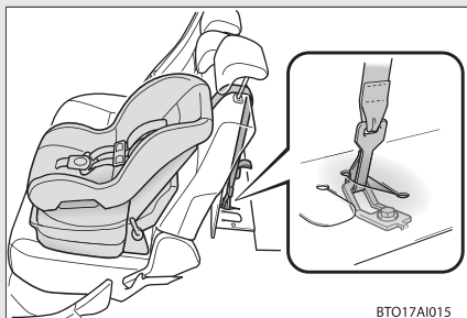
トップテザーアンカー (→ P. 81)
