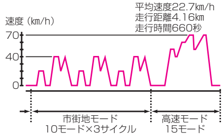
●図2. 「10・15モード」
