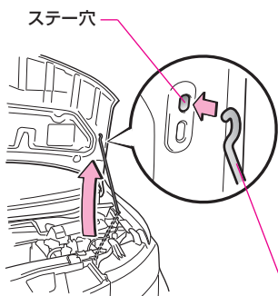
ボンネットステー
