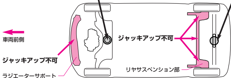
ガレージジャッキセット位置
